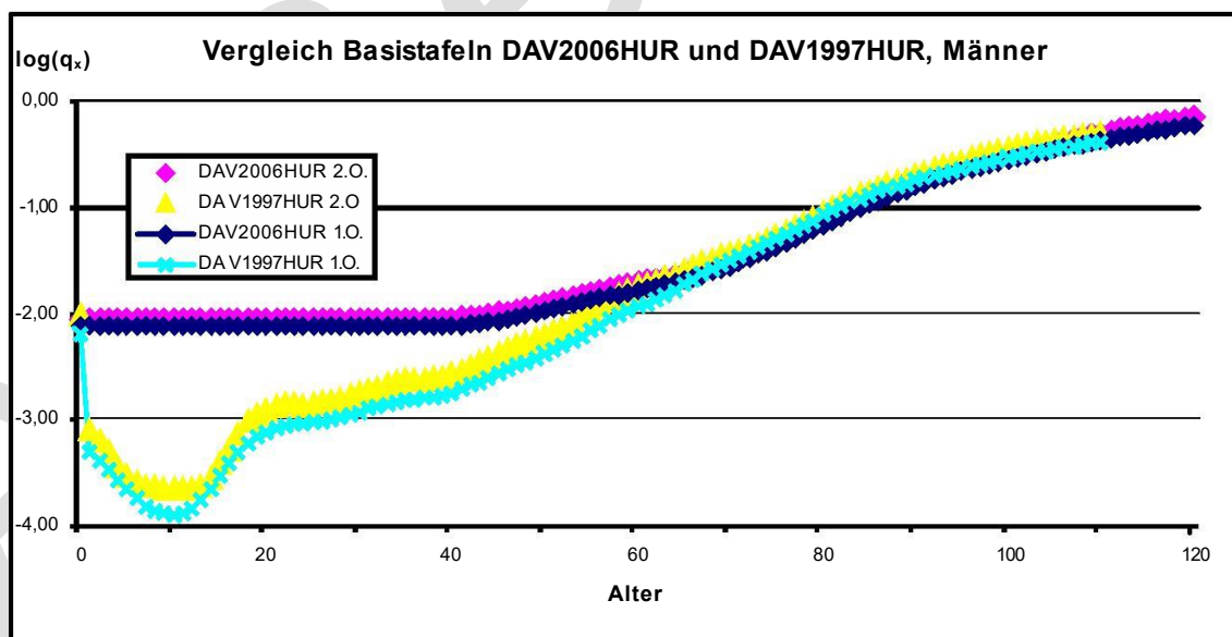
Abbildung 7: Vergleich der logarithmierten Basistafeln der DAV 2006 HUR und der DAV 1997 HUR sowohl erster als auch zweiter Ordnung, Männer.
